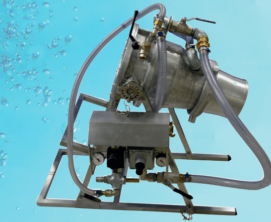
Das Inversions-Gerät ab DN 50 - 300...
